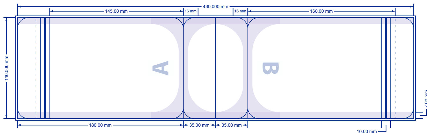
Příklad šablony - bez ventilu a eurozávěsu.
